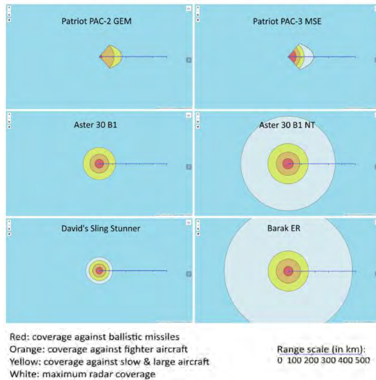
Εικόνα 8: Εκτιμώμενη κάλυψη πυραύλων ανάσχεσης (interceptor missile) 6 αντιαεροπορικών-αντιβαλλιστικών συστημάτων. Με κόκκινο χρώμα είναι η εκτιμώμενη κάλυψη εναντίον βαλλιστικών πυραύλων (TBM), με πορτοκαλί εναντίον μαχητικών Α/Φ και με κίτρινο εναντίον μεγάλων-αργών Α/Φ, κάλυψη η οποία συμπίπτει με την μέγιστη εμβέλεια. Με λευκό χρώμα αναπαρίστανται η κάλυψη του οργανικού ραντάρ του α/α συστήματος.
