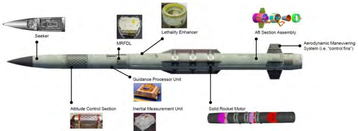
Εικόνα 5: Διάγραμμα του πυραύλου PAC-3 MSE ( https://f35.com/content/dam/lockheed-martin/mfc/documents/pac-3/24-09790-iamd-pac-3-mse-partner-ppt-updates_r2.pdf )
