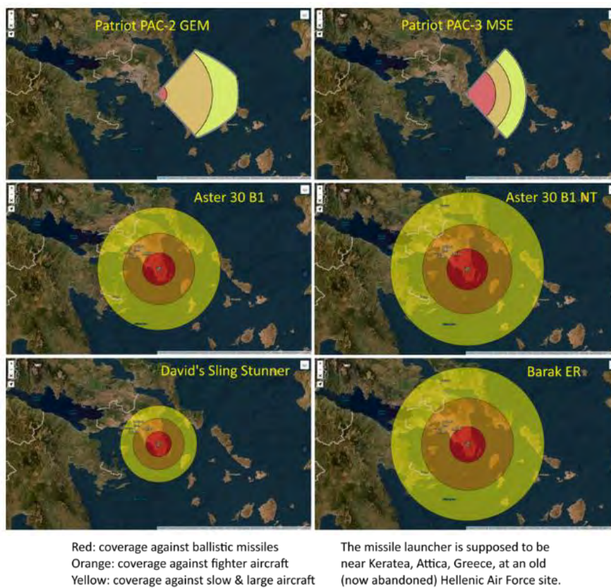
Εικόνα 9: Εκτιμώμενη κάλυψη πυραύλων ανάσχεσης 6 αντιαεροπορικών-αντιβαλλιστικών συστημάτων, τα οποία υποτίθεται ότι είναι τοποθετημένα στην "Πρώην Αεροπορική Βάση Κερατέας" (μία εγκαταλελειμμένη βάση της ΠΑ). Με κόκκινο χρώμα είναι η εκτιμώμενη κάλυψη εναντίον βαλλιστικών πυραύλων (TBM), με πορτοκαλί εναντίον μαχητικών Α/Φ και με κίτρινο εναντίον μεγάλων-αργών Α/Φ. Τα διαγράμματα έγιναν με τη βοήθεια του https://www.freemaptools.com/concentric-circles.htm .
