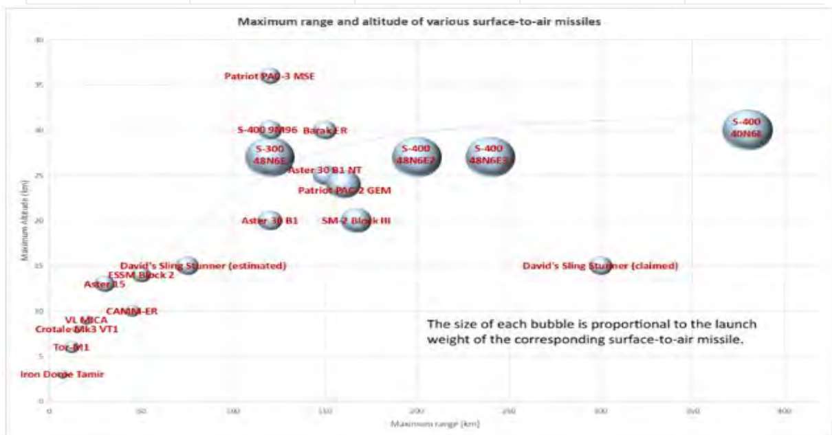
Εικόνα 14: Γραφική παράσταση μέγιστου ύψους και εμβείειας για διάφορους πυραύλους ανάσχεσης. Κάθε πύραυλος αναπαρίσταται ως μία σφαίρα, το μέγεθος της οποίας είναι ανάλογο του βάρους εκτόξευσης (launch weight).
