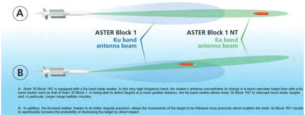
Εικόνα 7: Σύγκριση της δέσμης του ραντάρ του Aster 30 B1 με αυτήν του Aster 30 B1NT. Η υψηλότερη περιοχή συχνοτήτων Ka παρέχει πολύ πιο στενή δέσμη σε σχέση με την Ku και αναλόγως αυξημένη ακρίβεια, επιτρέποντας την επίτευξη άμεσης κρούσης (hit-to-kill). ( https://www.navalnews.com/naval-news/2024/10/first-test-firing-of-new-french-italian-aster-30-b1-nt-surface-to-air-missile/ )
