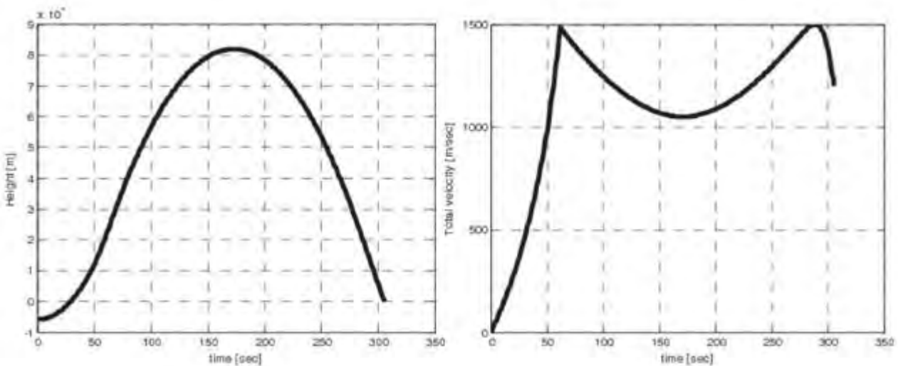
Εικόνα 3: Τυπική τροχιά (ύψος και ταχύτητα) συναρτήσει του χρόνου ενός τακτικού βαλλιστικού πυραύλου (TBM) με εμβέλεια 300 km ( https://ieeexplore.ieee.org/document/7244461 ). Ο πύραυλος επιταχύνει για τα πρώτα 60 s, φτάνοντας ταχύτητα 1500 m/s. Στη συνέχεια επιβραδύνει, συνεχίζοντας όμως την ανοδική του πορεία μέχρι το απόγειο, λίγο πάνω από τα 80 km. Από εκεί και πέρα, αρχίζει η πτωτική πορεία, αρχικά επιταχύνοντας. Σε ύψος γύρω στα 20 km, η πυκνότητα της ατμόσφαιρας είναι πλέον αρκετά υψηλή, με αποτέλεσμα να υπάρχει σημαντική επιβράδυνση. Όμως, ακόμα και μέχρι την πρόσκρουση, η ταχύτητα διατηρείται πάνω από 1200 m/s ή Mach 3,5. Εννοείται ότι για πυραύλους υψηλότερης κατηγορίας, η τερματική ταχύτητα είναι ακόμα μεγαλύτερη.
